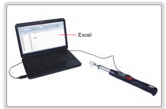
数据传输线(选配), 通过数据传输线输出键盘信号
